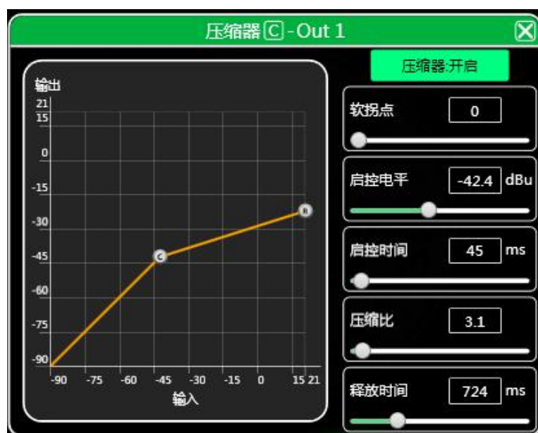
10.1 输出压缩器功能界面
