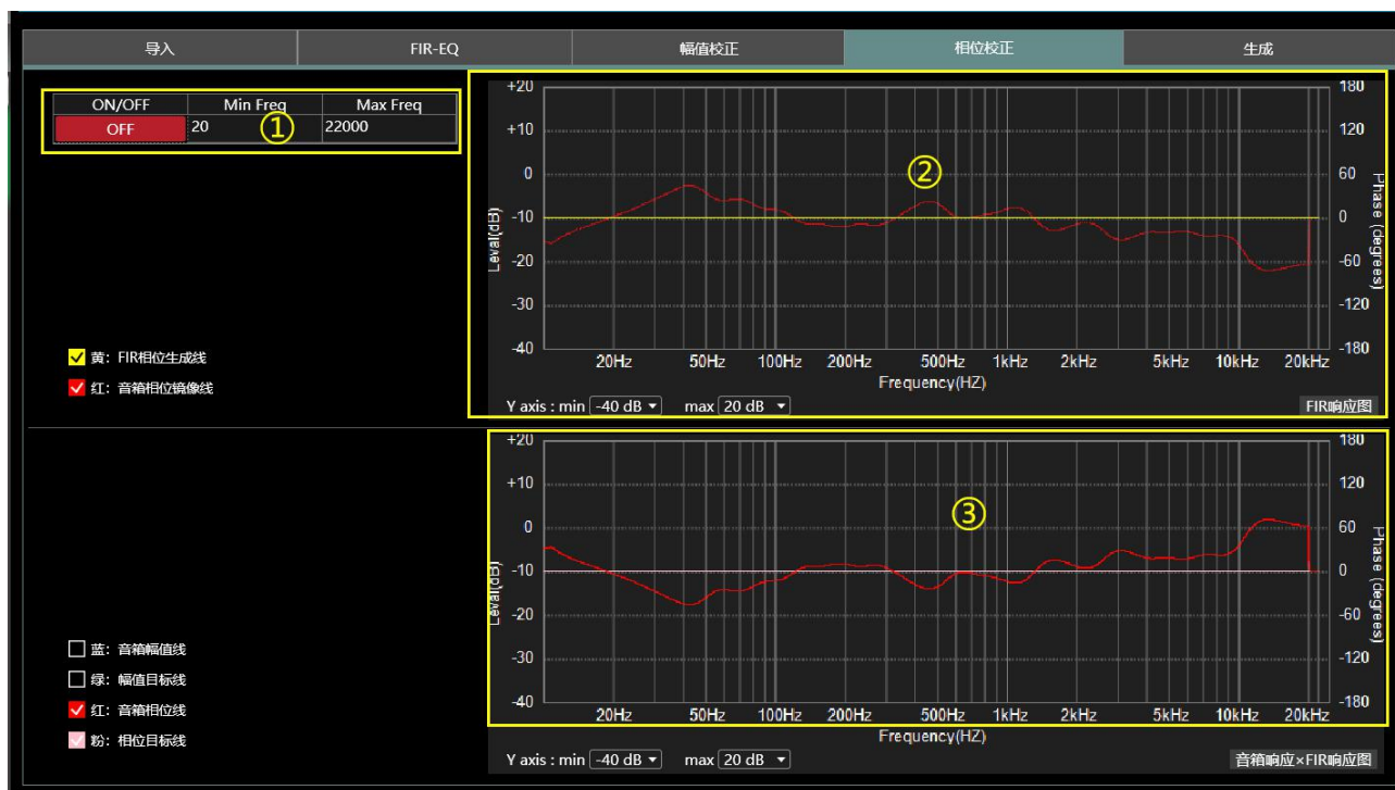
图 6.3 相位校正展示图
