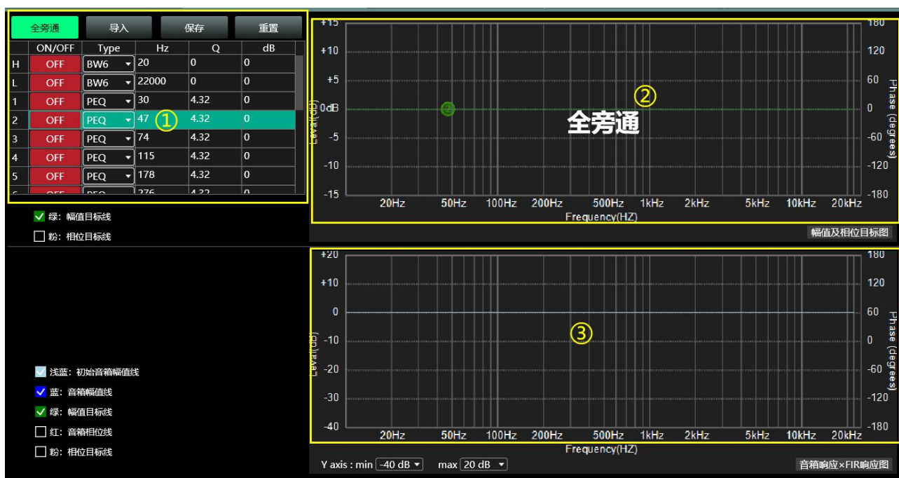
图 6.0FIR-EQ 设计界面
