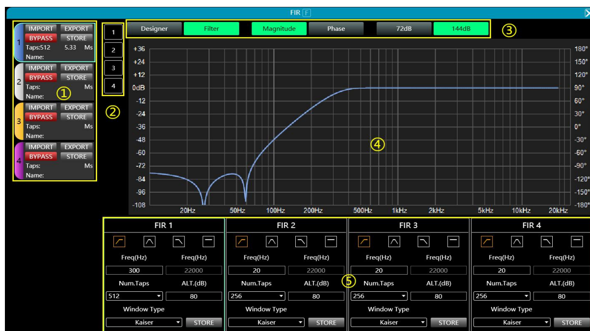
图 5.6 FIR 界面
