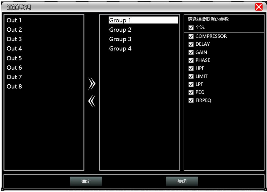
图 13.1 通道联调界面
