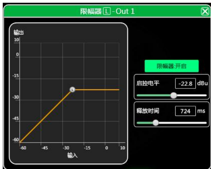
图 11.1 输出限幅器设置模块
